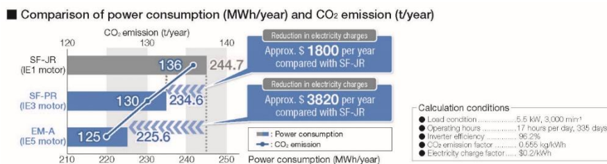
Bild 2: Energie- und CO 2 -Ausstoss Vergleich verschiedener Motorenarten
